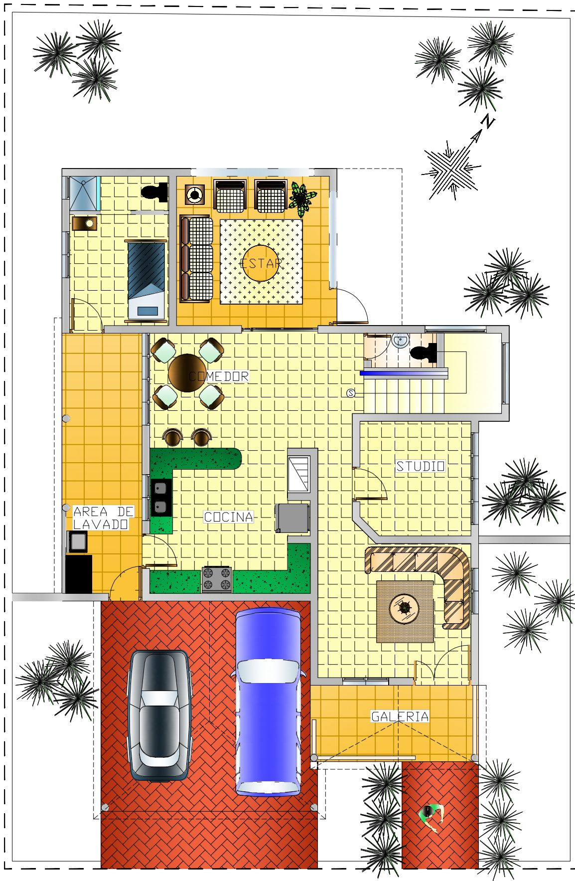
PLANTA ARQUITECTONICA AMUEBLADA I ER NIVEL
